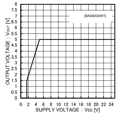
Fig.15 入力安定度 ( I_o=2A )
