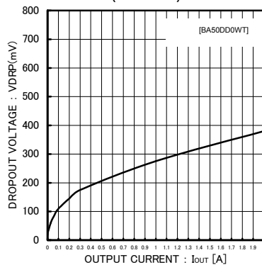
Fig.17 入出力電圧差 I_{OUT}-\Delta V_d 特性( V_{CC}=4.75V )
