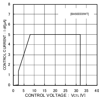
Fig.23 過電圧動作特性 ( I_o=200mA )
