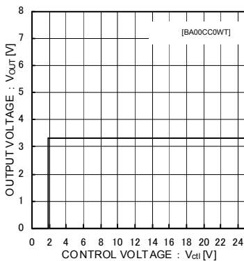
Fig.10 CTL 電圧 vs 出力電圧
