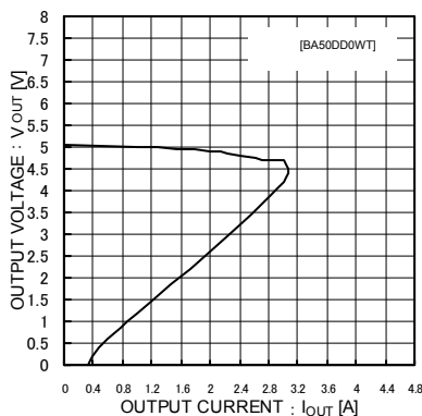
Fig.16 負荷安定度
