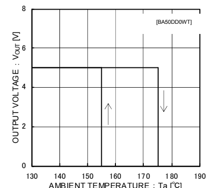
Fig.24 温度保護回路特性
