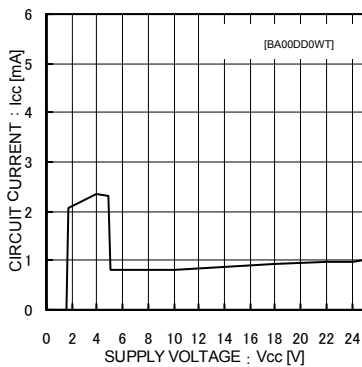
Fig.13 回路電流
