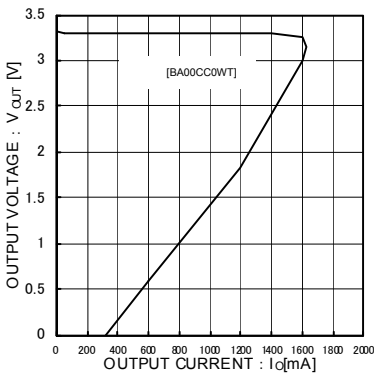
Fig.4 負荷安定度
