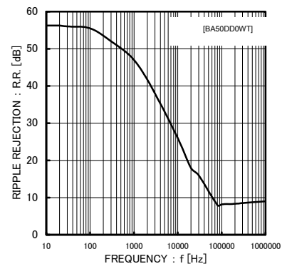
Fig.18 リップルリジェクション ( I_{out}=100mA )
