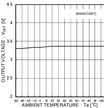
Fig.7 出力電圧温度特性
