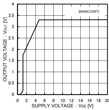
Fig.2 入力安定度
