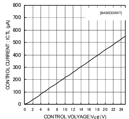
Fig.21 CTL 電圧 vs、CTL 電流
