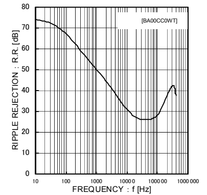
Fig.6 リップルリジエクション ( I_o=100mA )
