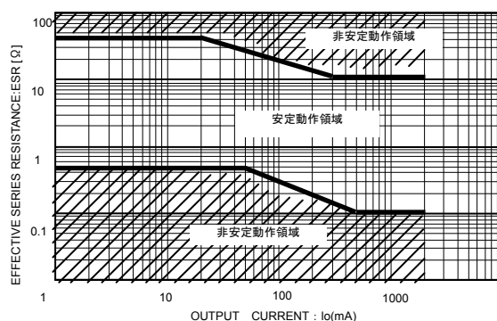
Fig.35 lo vs.ESR 特性(BA00DD0,22μF)
