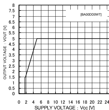
Fig.14 入力安定度 ( I_o=0mA )
