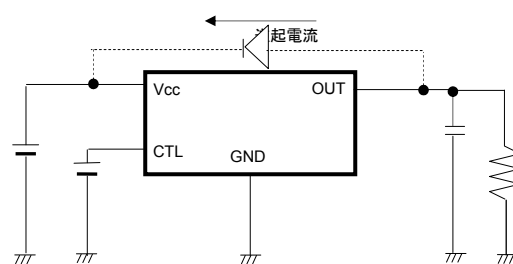
Fig.36 バイパスダイオード
