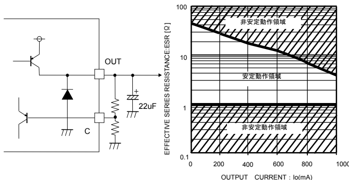
Fig.33 出力等価回路
