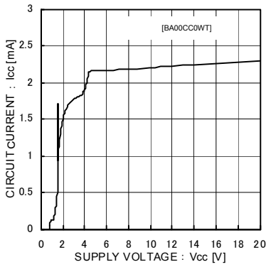
Fig.1 回路電流
