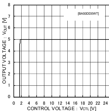
Fig.22 CTL 電圧 vs、出力電圧
